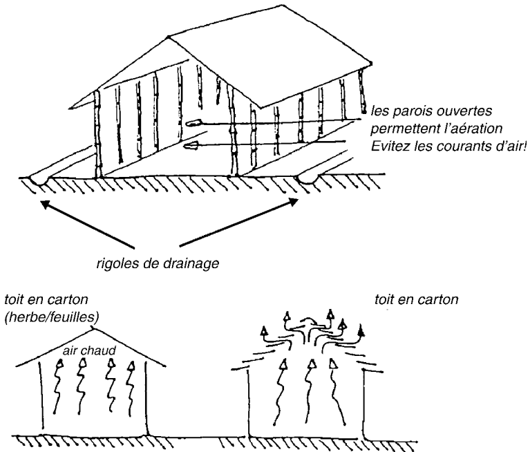
Figure 10 : Aération au moyen de parois et de toits ouverts
