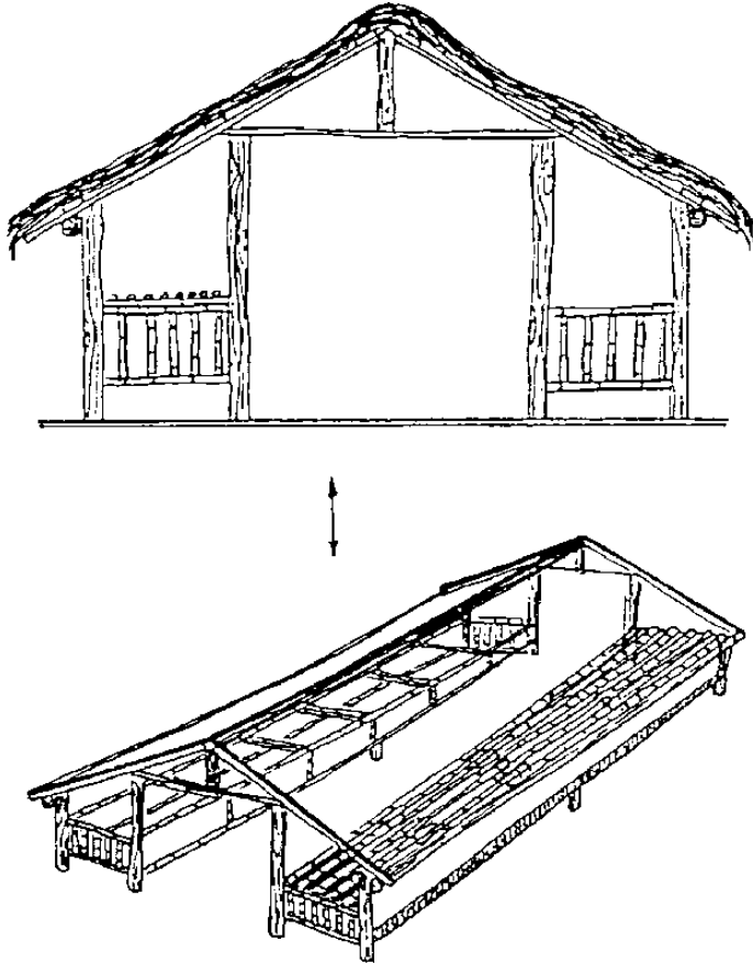
Figure 7 : Bâtiment d'élevage abritant 10 cages en bambou. Le toit est élevé et la construction bien aérée. Souvent utilisé sous les climats très chauds.
