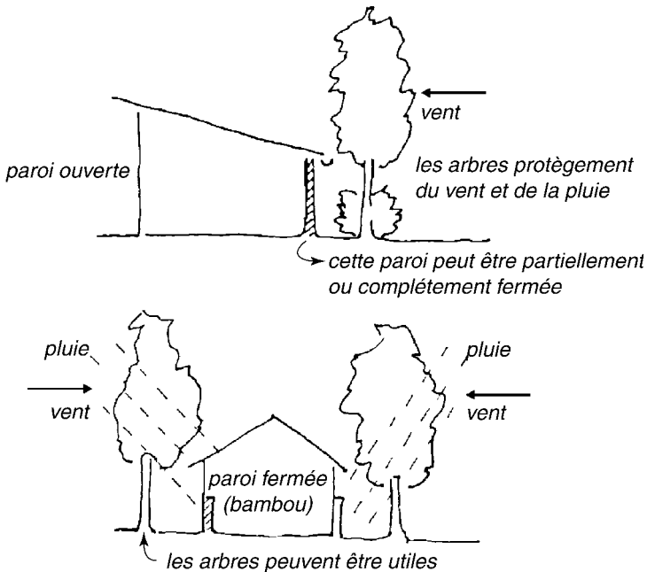
Figure 8 : Toit et arbres de protection contre la pluie et le soleil
