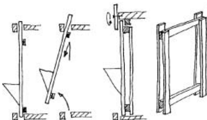
Figure 13 : Portes amovibles
